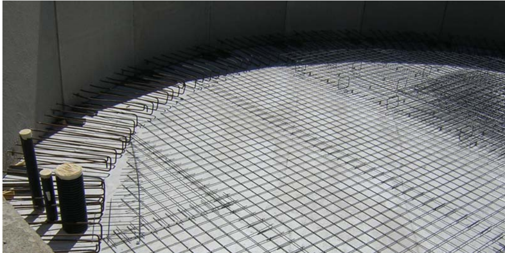
ARMADO Y HORMIGONADO DE SOLERA INTERIOR (A REALIZAR POR EL CLIENTE)
