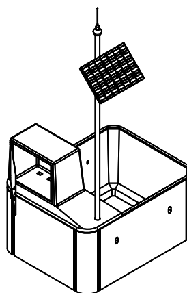
SOBREARQUETA NORMALIZADA PHA T-4 Y ARQUETA NORMALIZADA PHA T-4
