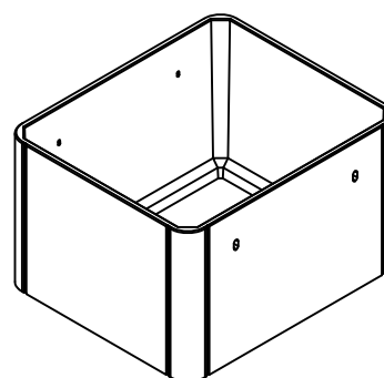
ARQUETA NORMALIZADA PHA T-7 (2.38x2x1.5)
