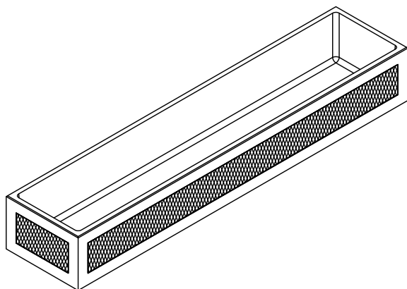
ABREVADERO PHA (5x1.1x0.7)
