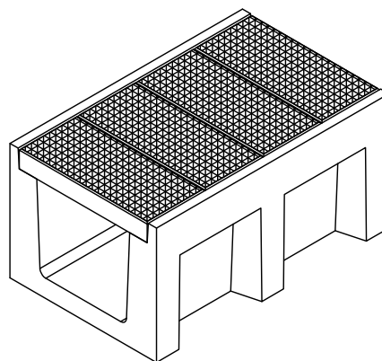
PASO CON LOSA PHA (0.74x0.7x2)
