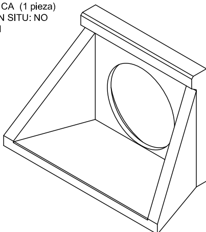
EMBOCADURA PHA C-100
