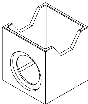
ARQUETA DRENAJE (1x1x1.1)
