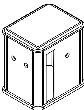
CASETA NORMALIZADA PHA T-4 (GENERADOR) (2x1.5x2.25)
