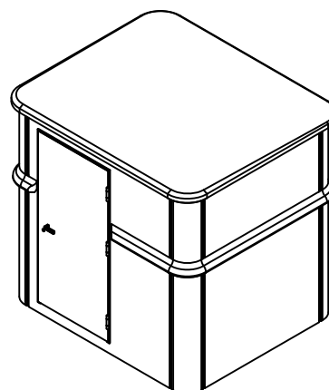
CASETA NORMALIZADA PHA T-7 (2.38x2x2.4)
