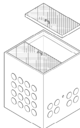
ARQUETA CT (90x90x115)
